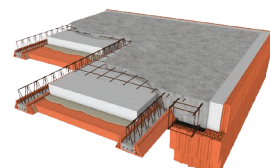
Stropný systém HURDIS
