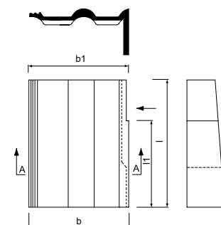
BOČNÍ POHLED
