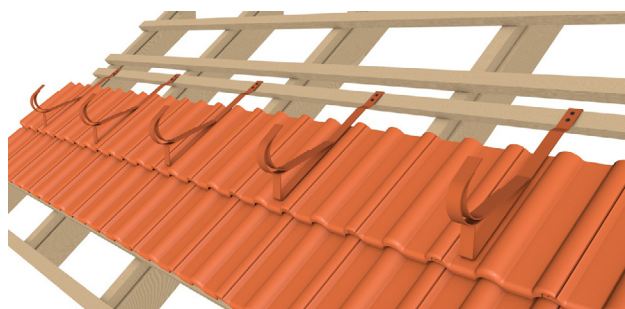
Přídavná lať 40/60, 3x vrut \varnothing 5 mm
