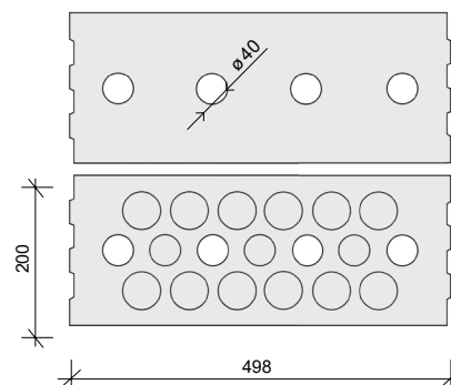
Převazba rohu 200/200 mm 14DF/14DF
