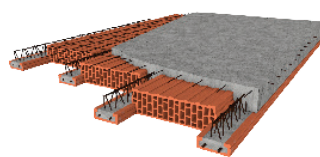
Stropný systém MIAKO
