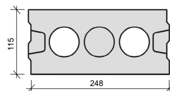
Vazba rohu z 4DF-LDE Roh vnitřní stěny tl. 115 mm
